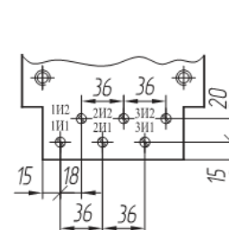
Трансформаторы с вторичными обмотками от одной до трех
