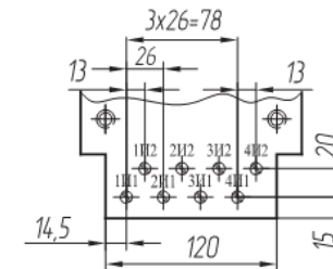
Трансформаторы с вторичными обмотками от одной до четырех
